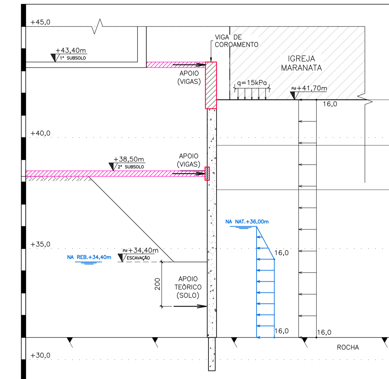
DETALHE 14.6B: CORTINA DE ESTACAS SECANTES IGREJA MARANATA FASE PROVISÓRIA 02
