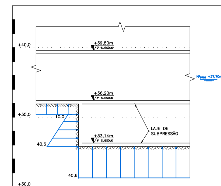
DETALHE 14.4: SUBPRESSÃO NAS LAJES DO 3º E 4º SUBSOLO
