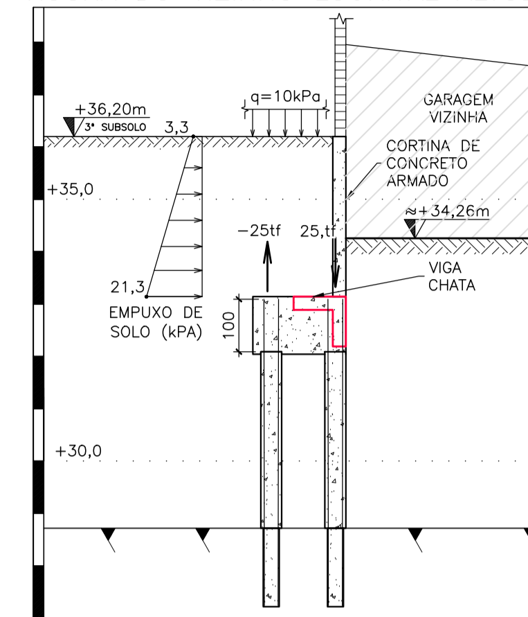
DETALHE 14.3: CONTENÇÃO APOIADA SOBRE BLOCOS DE ESTACAS RAÍZ ANCORADAS NA ROCHA DO VIZINHO LOURIVAL ALTOÉ
