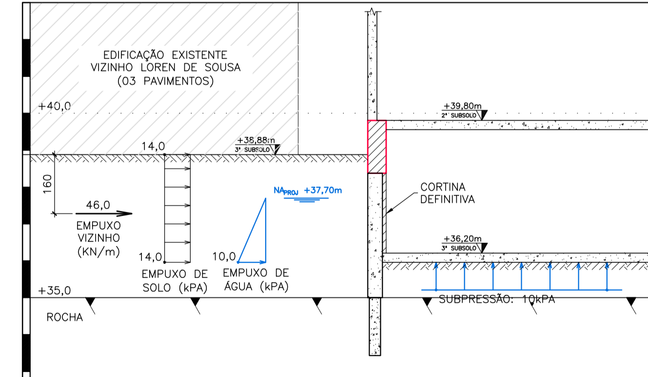
DETALHE 14.2B: CORTINA DE CONCRETO ARMADO CONVENCIONAL DOS VIZINHOS LOREN E NILDON FASE DEFINITIVA
