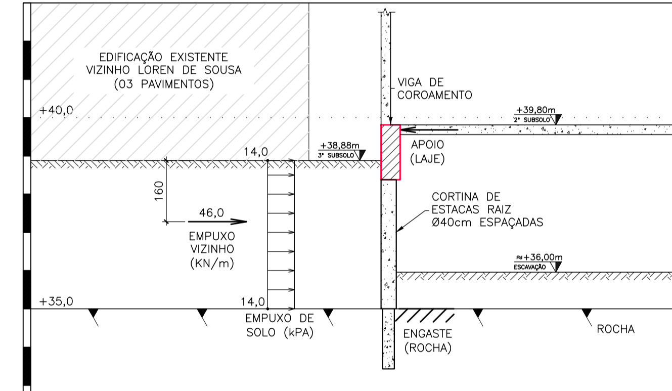
DETALHE 14.2A: CORTINA DE ESTACAS RAÍZ ESPAÇADAS DOS VIZINHOS LOREN E NILDON DE SOUSA FASE PROVISÓRIA
