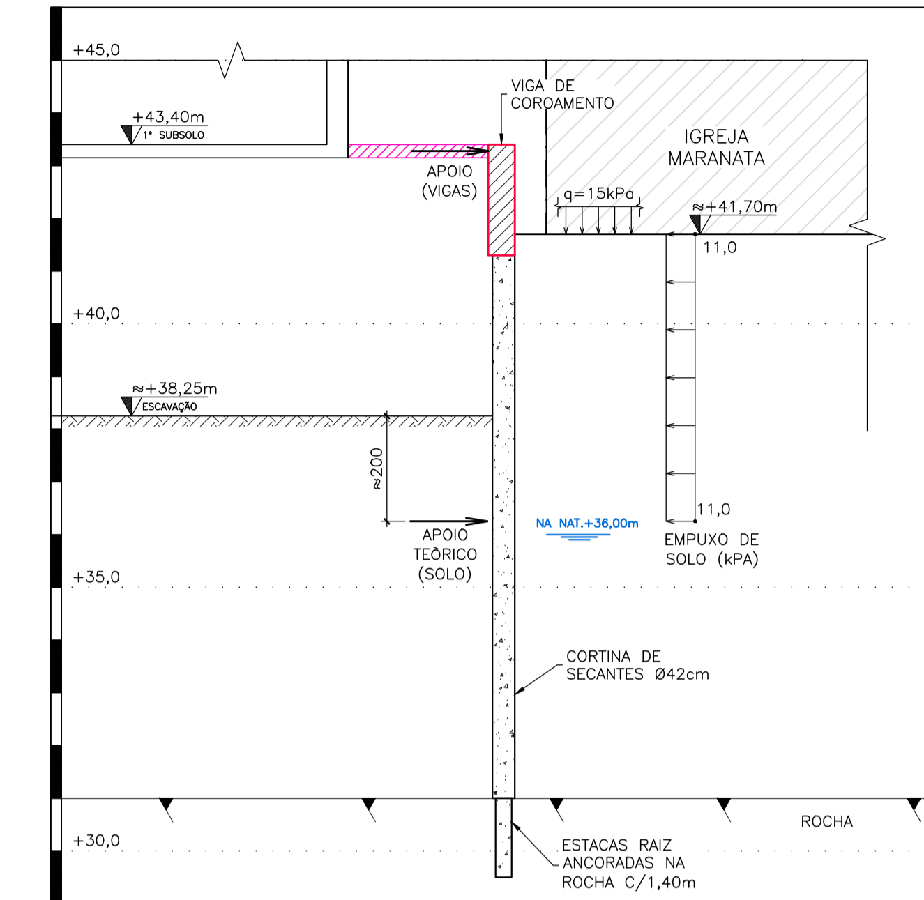
DETALHE 14.6A: CORTINA DE ESTACAS SECANTES IGREJA MARANATA FASE PROVISÓRIA 01
