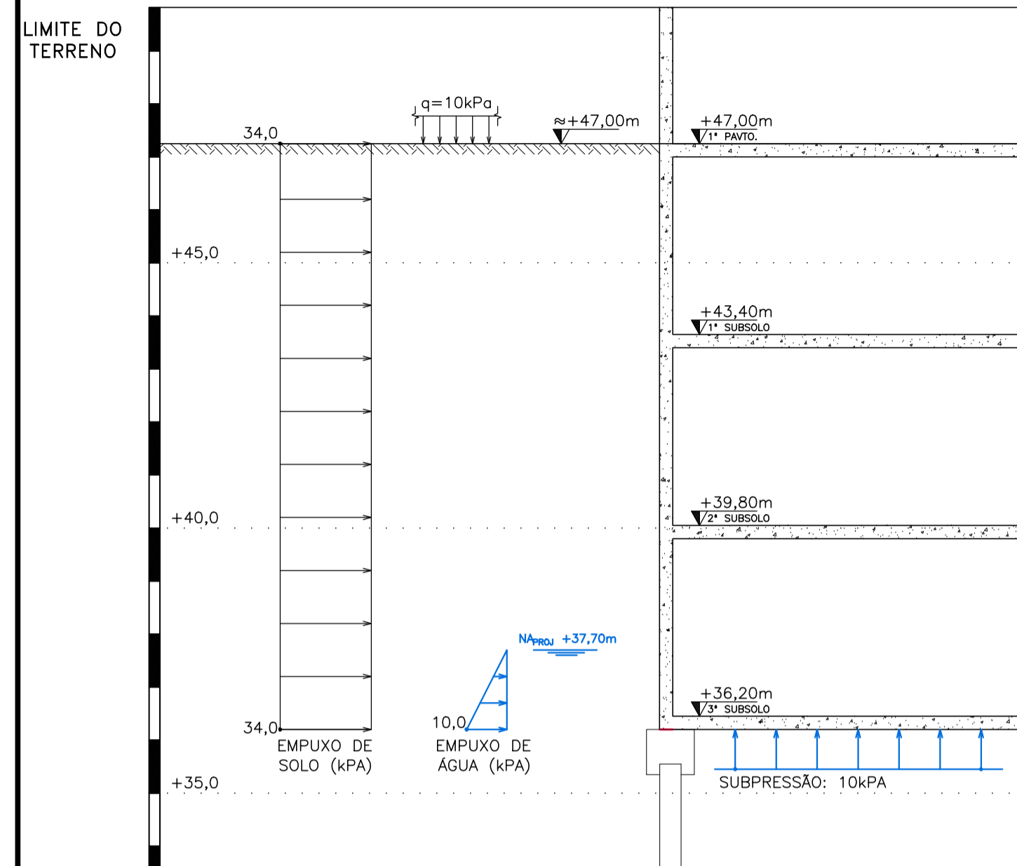
DETALHE 14.1: CORTINA DE CONCRETO ARMADO CONVENCIONAL DA RUA HONORINA DE OLIVEIRA
