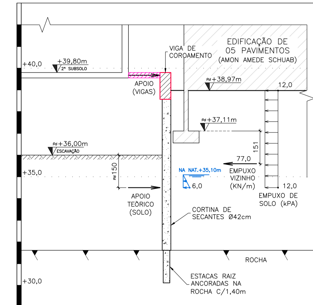
DETALHE 14.5B: CORTINA DE ESTACAS SECANTES DO VIZINHO AMON SHUAB FASE PROVISÓRIA 02
